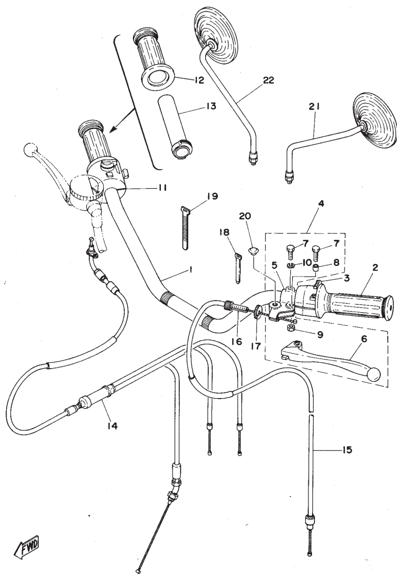
Fig. 25 HANDLE · WIRE
