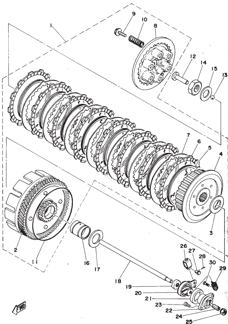
Fig. 5 CLUTCH
