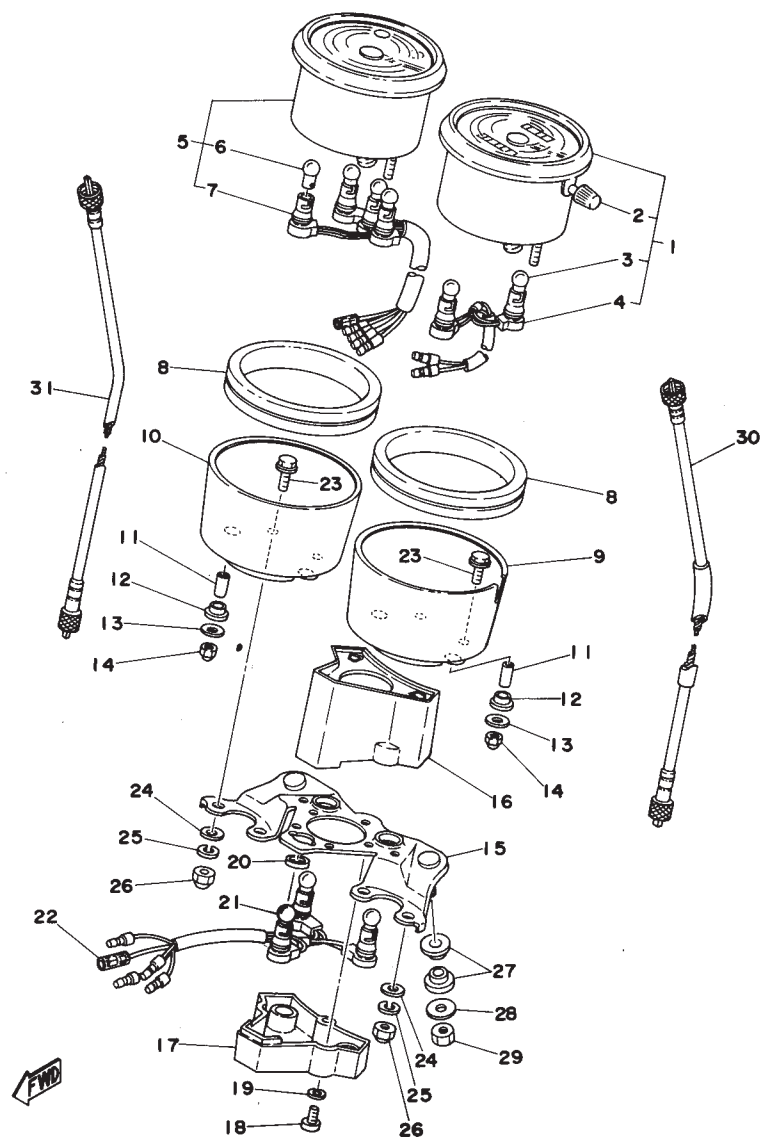
Fig. 42 SPEEDOMETER · TACHOMETER
