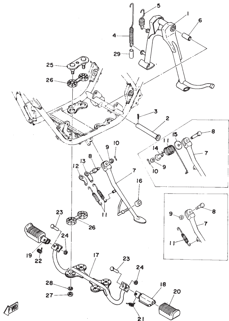
Fig. 19 STAND · FOOTREST
