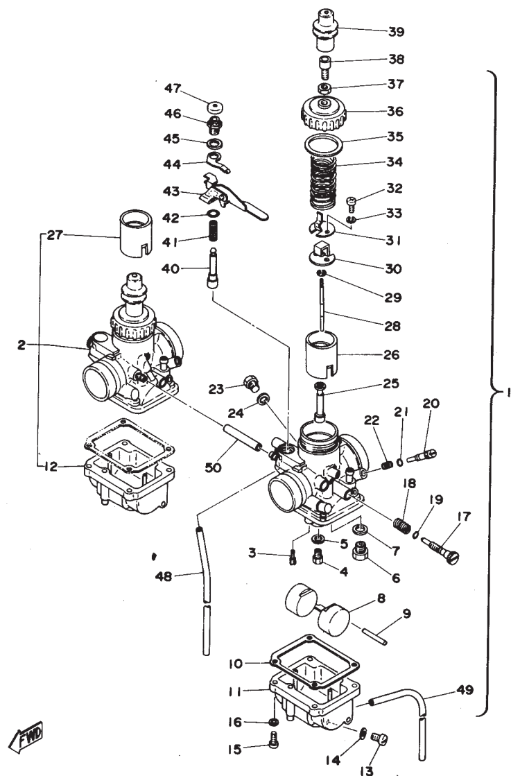
Fig. 12 CARBURETOR
