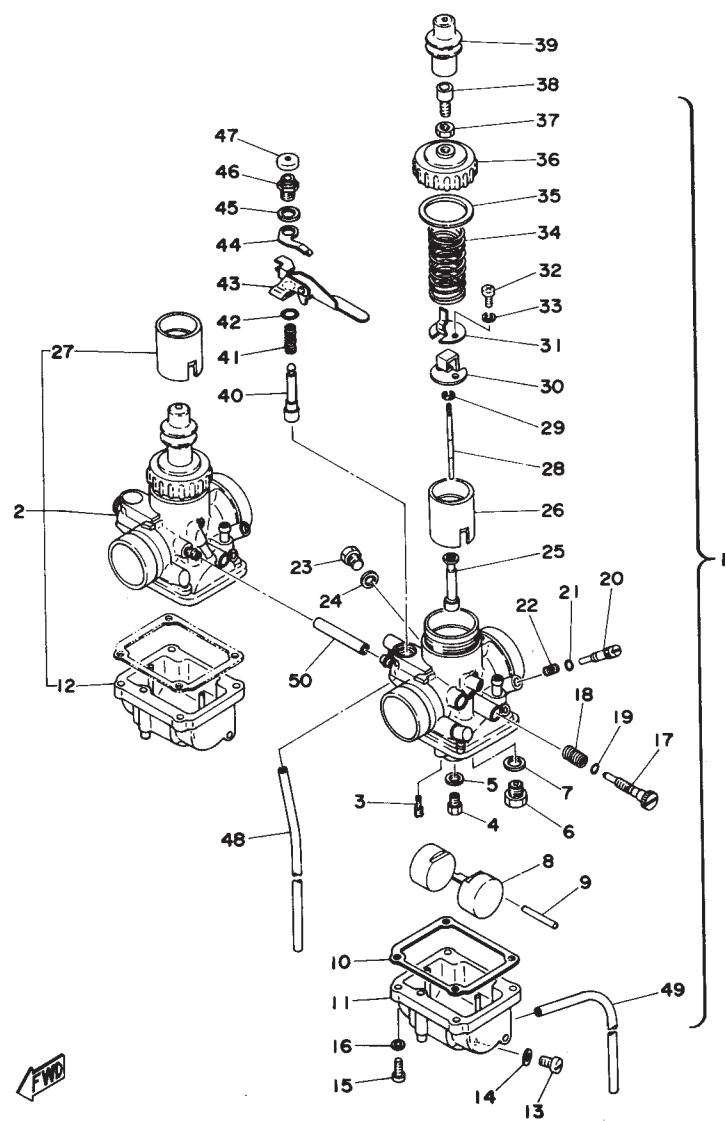
Fig. 12 CARBURETOR
